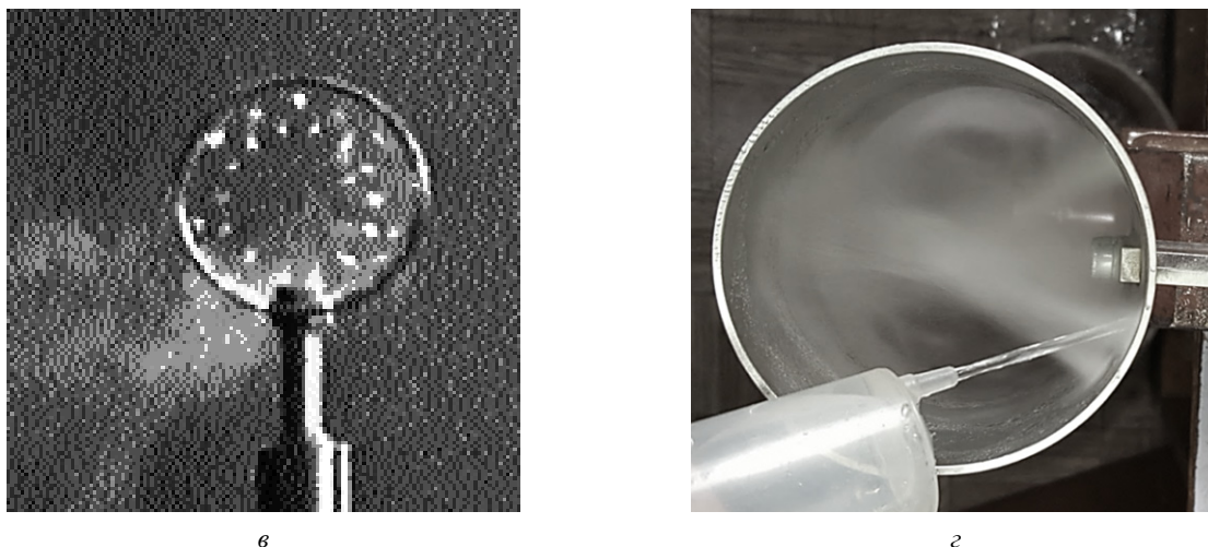
Рис. 10. Результаты экспериментальных исследований работы ультразвукового трубчатого вибратора при осушении воздуха: а – визуализация ультразвукового поля при радиальных колебаниях вибратора; б, в – визуализация ультразвукового поля при радиально-изгибных колебаниях вибратора; г - процесс ультразвукового разпиления у тонкому шарі
