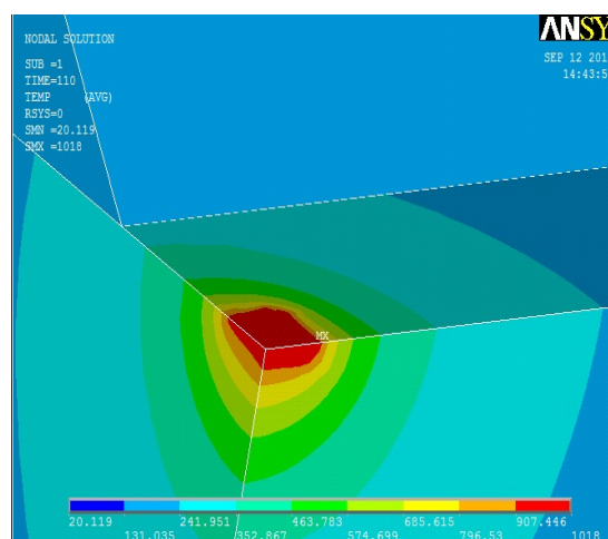
Рис. 3. Розподіл температури різання по контактним ділянкам різця в процесі моделювання
