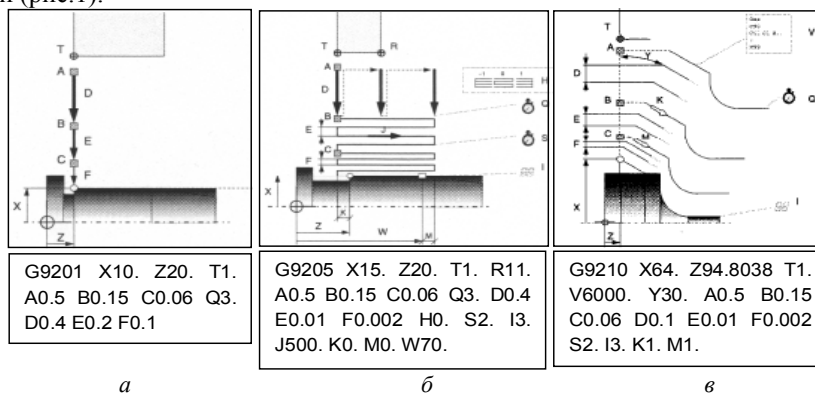
Рис. 1. Схемы операций шлифования и примеры циклов: а – врезное шлифование; б – продольное шлифование; в – контурное шлифование
