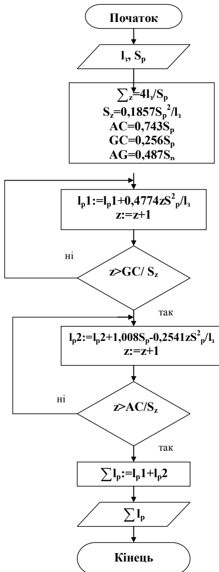
Рис. 2. Структурна схема алгоритму для розрахунку сумарної довжини різальних кромок гребінок \sum l_p та подачі на зуб S_z
