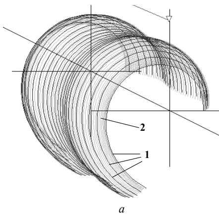
Рис. 8. Результати контролю: а – сітки заданої і вимірної форм, б – розподіл похибки за формою ендопротезу
