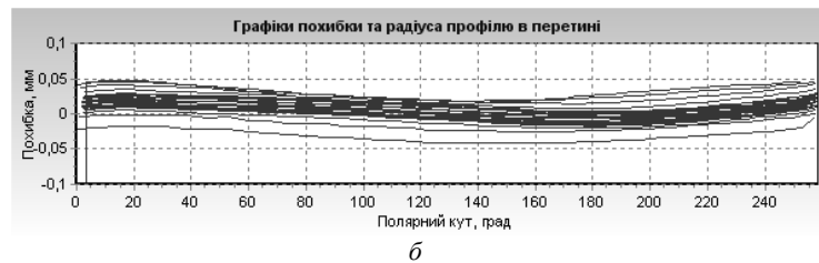
Рис. 8. Результати контролю: а – сітки заданої і вимірної форм, б – розподіл похибки за формою ендопротезу
