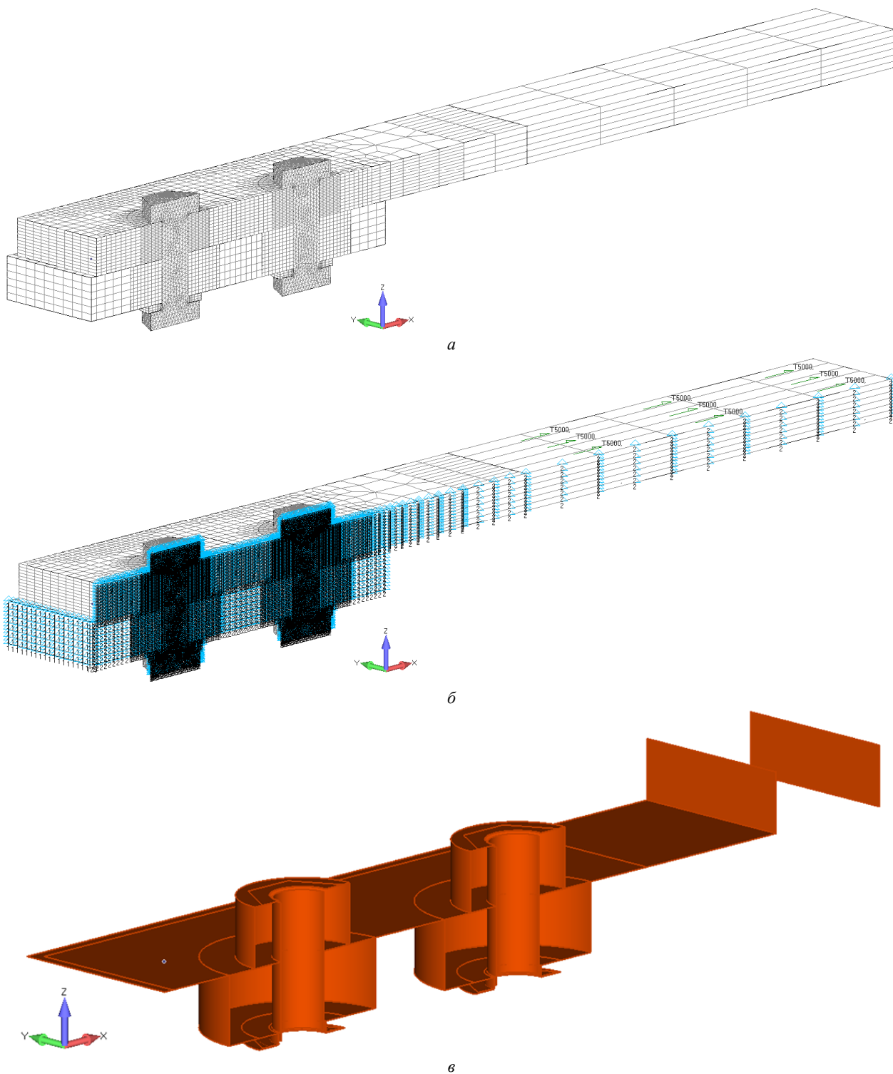
Рис. 3. Змішана скінченно-елементна модель зразка однозрізного болтового з'єднання з ПКМ: а – скінченно-елементна модель; б – скінченно-елементна модель з умовами обмежень переміщень у вузлах та сило- вим навантаженням; в – призначені поверхні "склеювання" та можливого контакту (Connectors)
