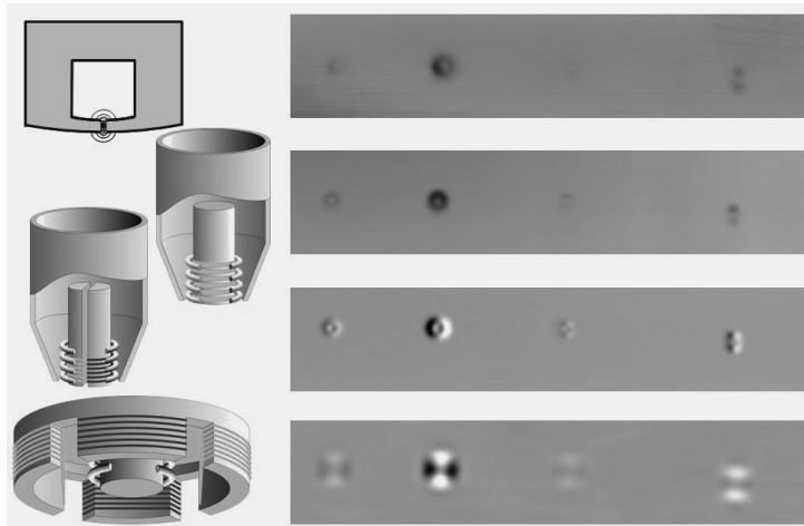
Bild 2. Wirbelstromsensoren und deren Abbildungseigenschaften an TiAl6V4. Links: Spaltsensor, koaxialer Absolutsensor, Differenzsensor, Multidifferenzsensor. Rechts: Wirbelstromsignale dieser Sensoren an Bohrungen mit 0,4 und 0,8 mm Durchmesser und Schlitzen der Länge 0,4 und 0,8 mm mit Tiefen von 0,2 und 0,4 mm
