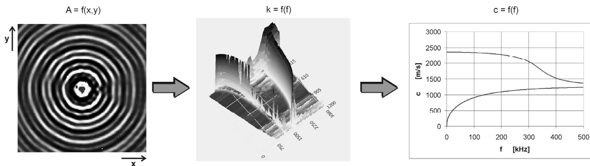
Bild 13. Verarbeitung von Wellenfelddaten zu Dispersionsdiagrammen
