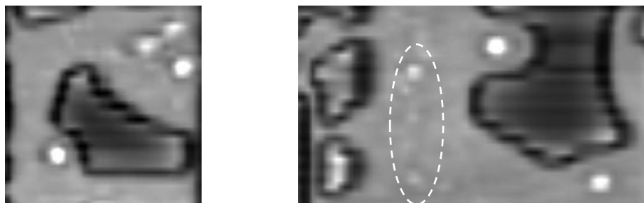
Bild 9. Wirbelstrombilder offener und verdeckter Poren in Aluminiumdruckguss
