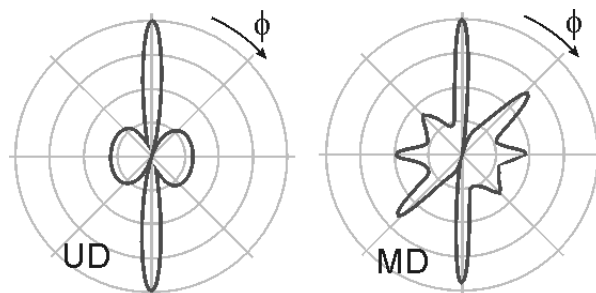
Bild 5. Polardiagramme kolinearer Wirbelstromsensoren zeigen die Anisotropie der Leitfähigkeit von unidirektionalem (UD) und multidirektionalem (MD) CFK
