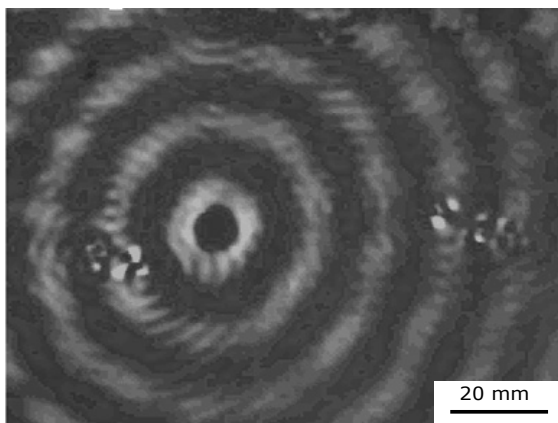
Bild 14. Wechselwirkung von Lamb-Wellen mit Impactschäden
