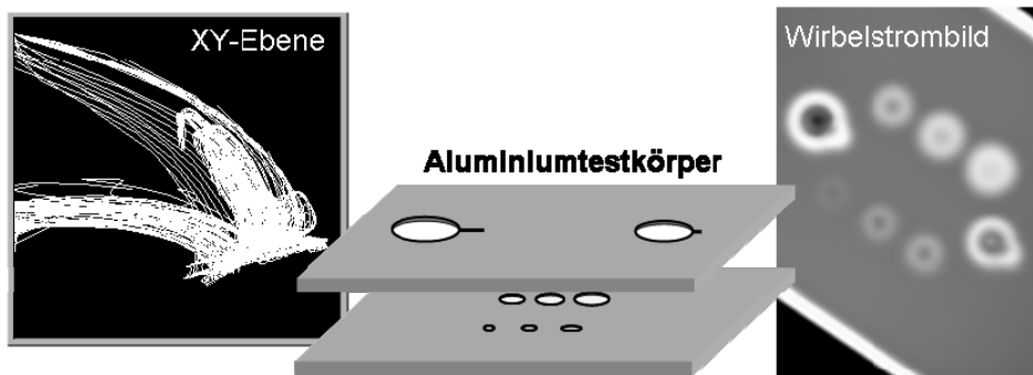
Bild 7. Wirbelstromsignale eines zweilagigen Aluminium-Testkörpers
