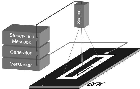
Bild 12. Scanning-Laser-Vibrometer-Messsystem
