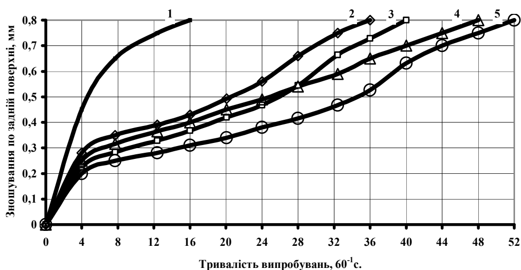
Рис. 2. Кінетика зношування БНТП зі сплаву ВК8 з різними покриттями при точинні сталі 12X18Н10Т 1-без покриття; 2- TiC; 3- TiC, TiN; 4- MAO+TiC+MAO; 5- MAO+(TiC, TiN)+MAO v = 2,5\text{м/с} ; s = 0,434\text{ мм/об} ; t = 1,0\text{ мм}
