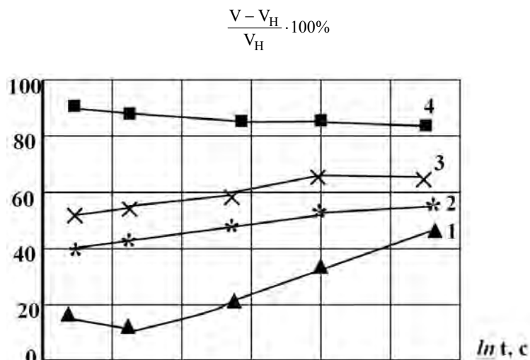
Рис. 3. Зміни швидкостей релаксації напружень V після витримки зразків у різних середовищах порівняно з швидкостями релаксації контрольних зразків V_H . 1 - дистильована вода; 2 - сольовий розчин; 3 - рідина СЖР-3; 4 - гальмівна рідина
