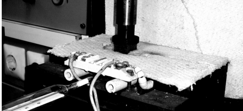
Рис. 1. Пристрій для вимірювання в'язко-пружних характеристик гальмівних колодок
